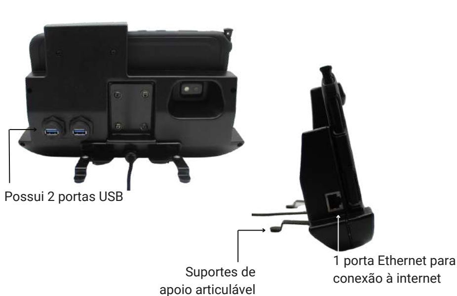
Doca de mesa para tablet Samsung Active 3 e Active 5 Código: DCK040005
