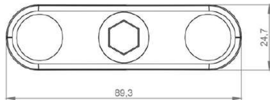
Brazo corto Tamaño B (1") Código: BRC040003 Peso: 80 g
