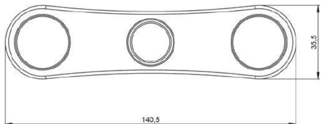
Brazo largo Tamaño C (1,5") Código: BRC040002 Peso: 160g
